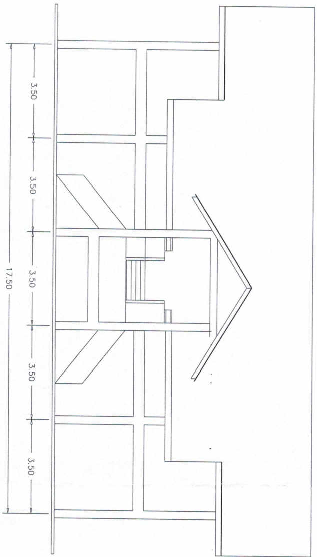
รูปด้านหน้า 1:100
